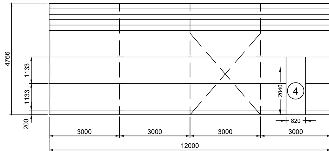
1 RIGHT ELEVATION 3 SCALE: 1:100
