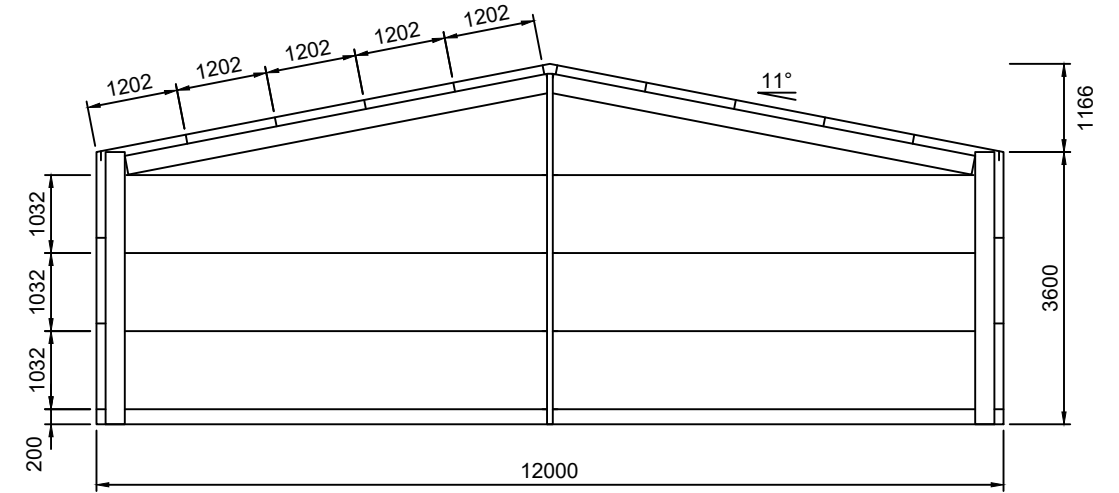
3 REAR ELEVATION 3 SCALE: 1:100 FRAME #5
