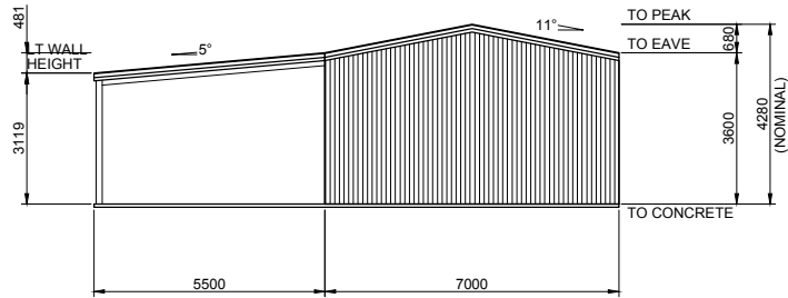
3 ENDWALL EXTERIOR ELEVATION 7 SCALE: 1 = 200
