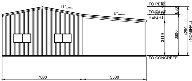
4 ENDWALL EXTERIOR ELEVATION 7 SCALE: 1 = 200
