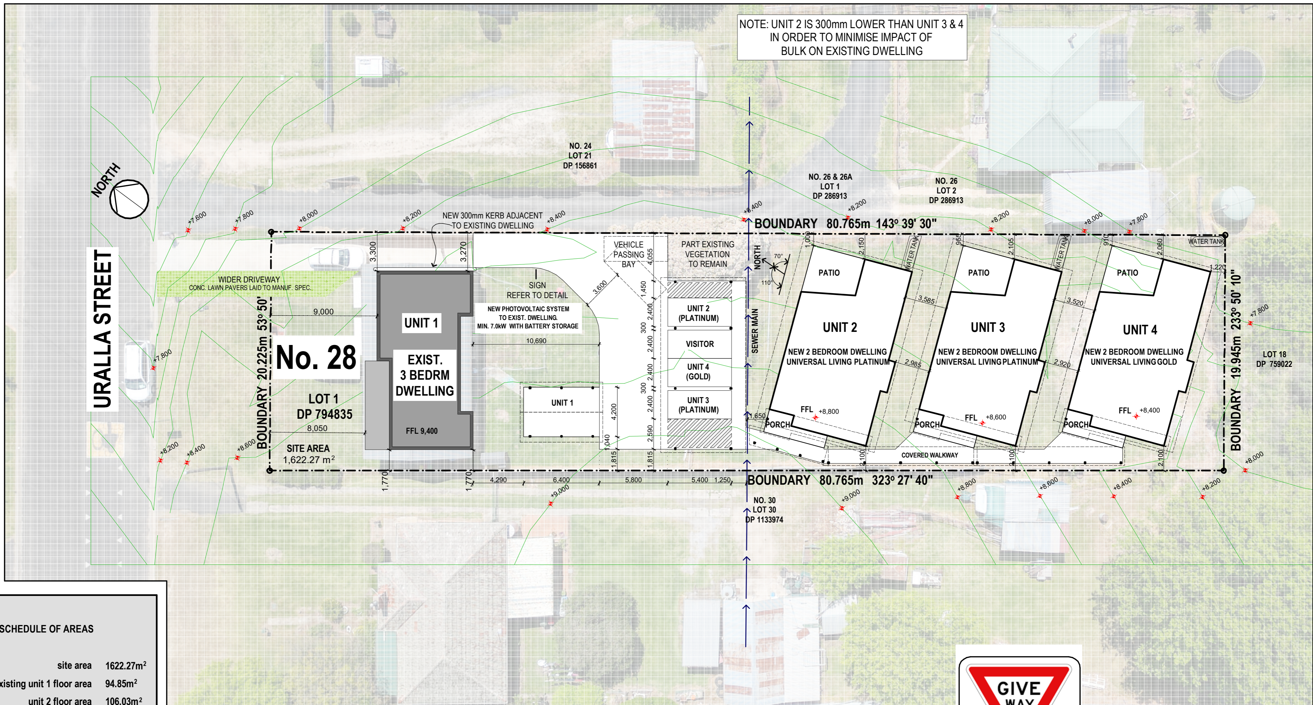
SITE PLAN 1:200
