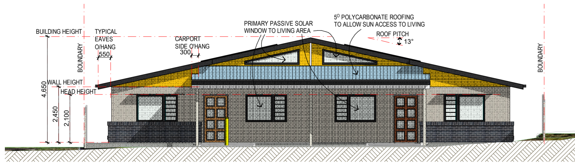
N ELEVATION 1:100
