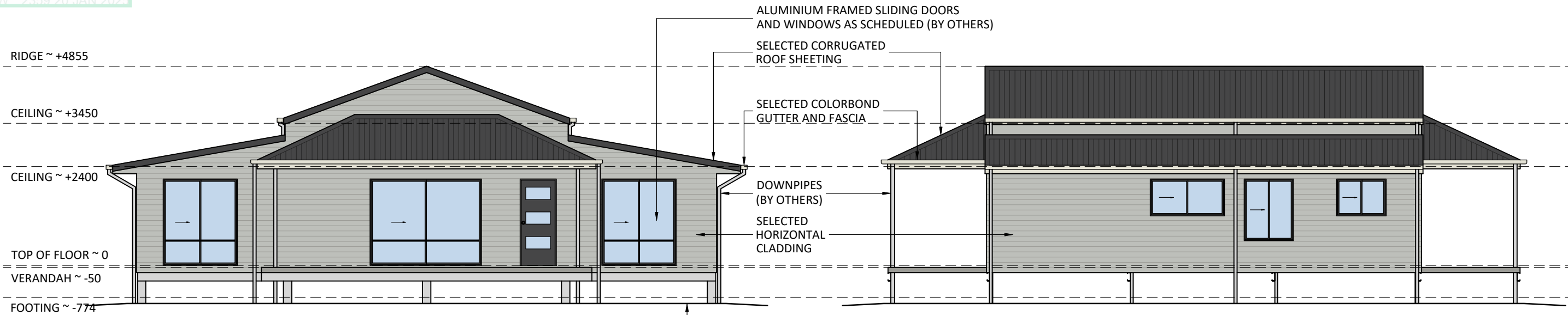
ELEVATION 1
