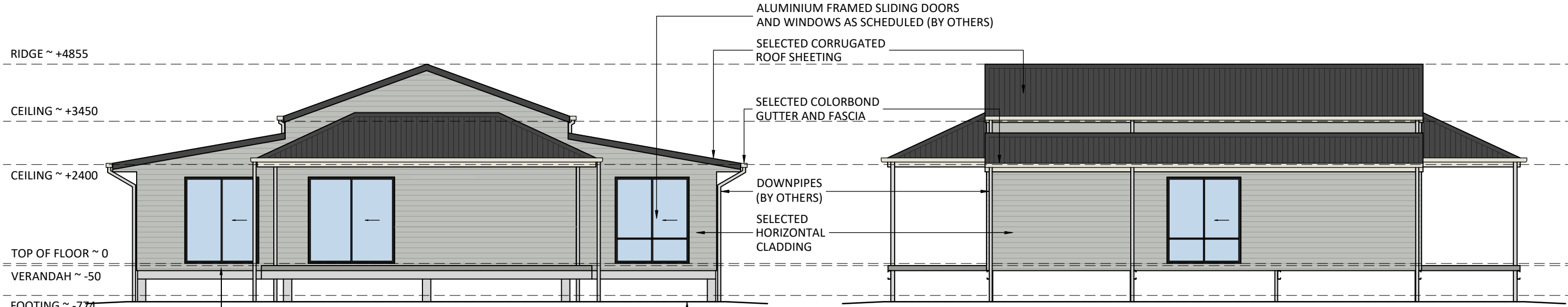
ELEVATION 3
