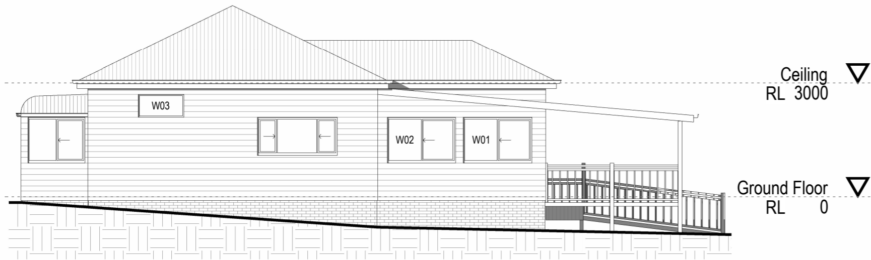
1 NE Elevation 1 : 100
